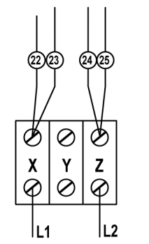
480 VOLT 1 PHASE
