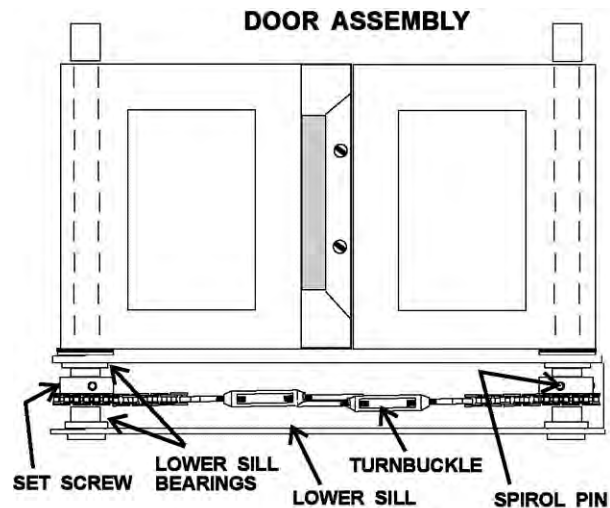
DOOR ASSEMBLY
