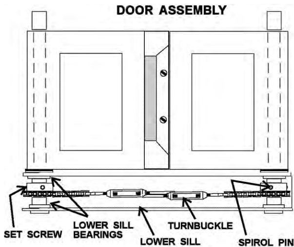
DOOR ASSEMBLY
